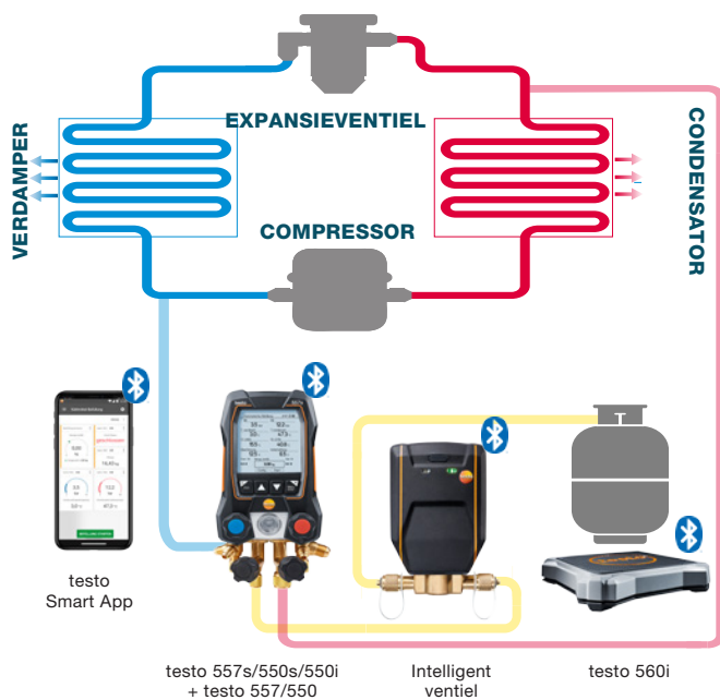
Schema voor automatische koelmiddelvulling
